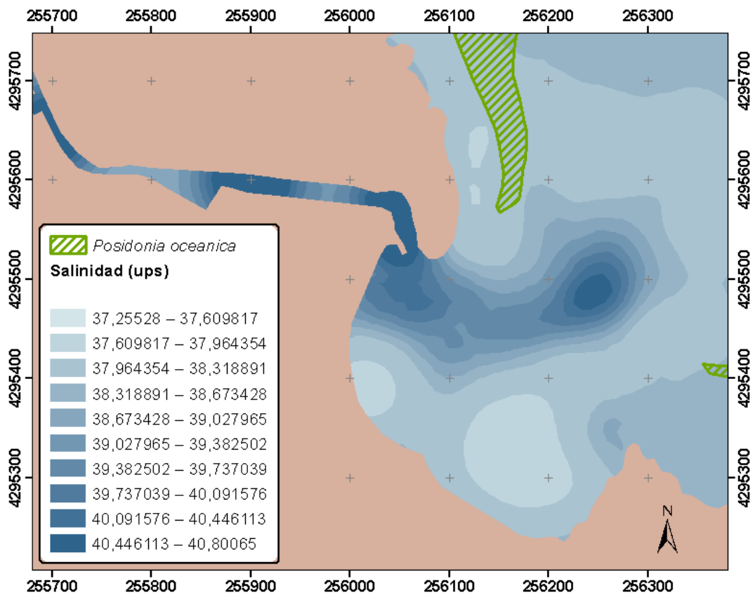
Figura 3: Distribución de la salinidad en el fondo
